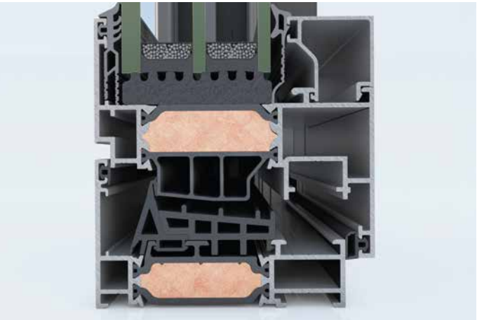
ELVIAL I² _ ΚΑΙΝΟΤΟΜΟΣ ΤΕΧΝΟΛΟΓΙΑ ΜΟΝΩΣΗΣ ΑΦΡΩΔΕΣ ΘΕΡΜΟΜΟΝΩΤΙΚΟ ΠΡΟΦΙΛ ΕΛΑΣΤΙΚΑ ΜΕ ΠΤΕΡΥΓΙΑ
